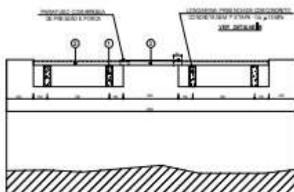
CORTE TRANSVERSAL B - B SÍMBOLO
